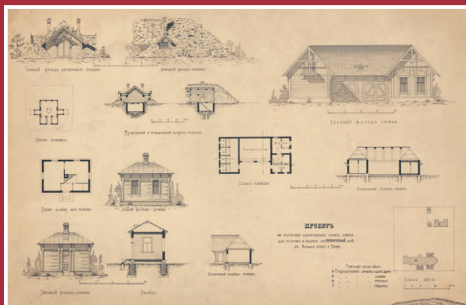
Проект на постройку деревянных служб, домика для сторожа и ледника при архиерейской даче в Курьях. Начало XX века.
