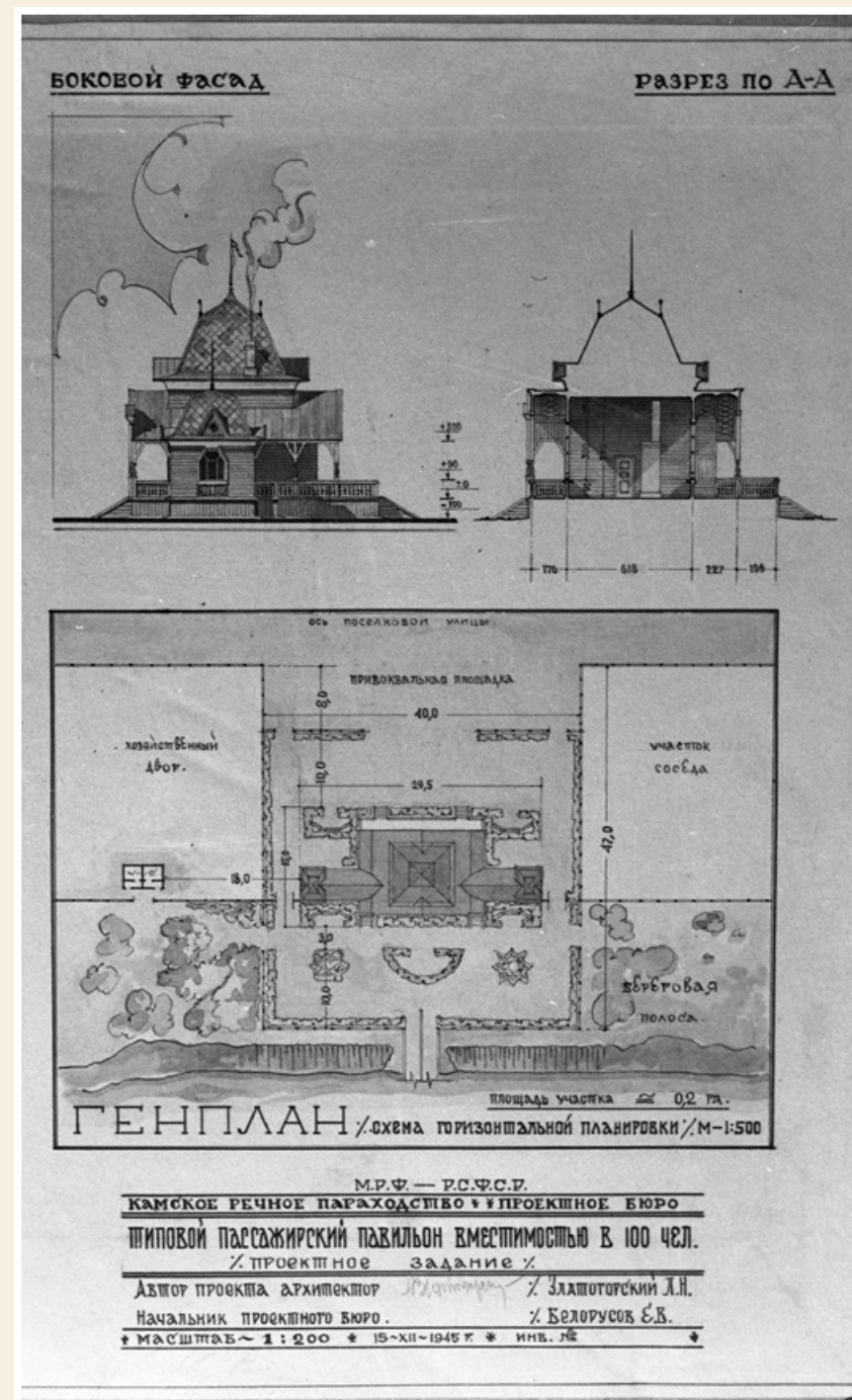
Типовой проект пассажирского павильона вместимостью 100 человек. Автор проекта — архитектор Л. Н. Златогорский, проектное бюро Камского речного пароходства. 1945 г. Фотокопия. ГАПК. Ф. р-1619. Оп. 1. Д. 24. Л. 4.
