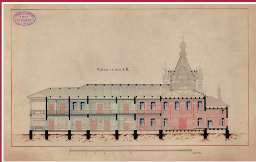
Чертёж продольного разреза здания архиерейской дачи в Курьинских дачах, выполненный архитектурно-строительным бюро А. Б. Турчевича в г. Перми. Начало XX века. Подлинник. Рукопись. ГАПК. Ф. 716. Оп. 1. Д. 665.
