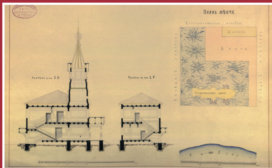
План местности и чертёж продольного разреза здания архиерейской дачи в Курьинских дачах, выполненный архитектурно-строительным бюро А. Б. Турчевича в г. Перми. Начало XX века.
