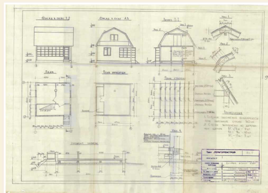
Проект дачного домика 6×6 м треста «Пермгорремстрой». 1982 г. Копия. Рукопись. ГАПК. Ф. р-214. Оп. 7. Д. 47. Л. 97.
