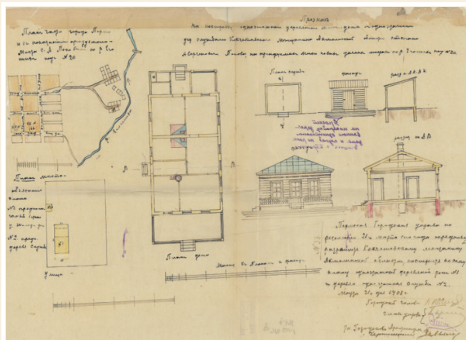
План дачного места и проект на постройку одноэтажного деревянного жилого дома с деревянными службами Кочетковского мещанина Акмолинской области С. А. Попова на арендуемых дачных местах по речке Егошихе под № 20. 1908 г. Подлинник. Рукопись. ГАПК. Ф. 716. Оп. 1. Д. 746.
